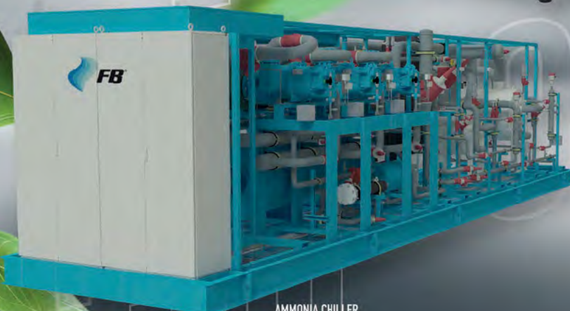
AMMONIA CHILLER
